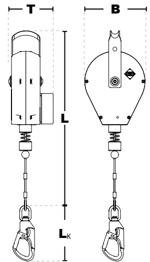
IKV 21 (EN 362:2004) mit Fallanzeiger
