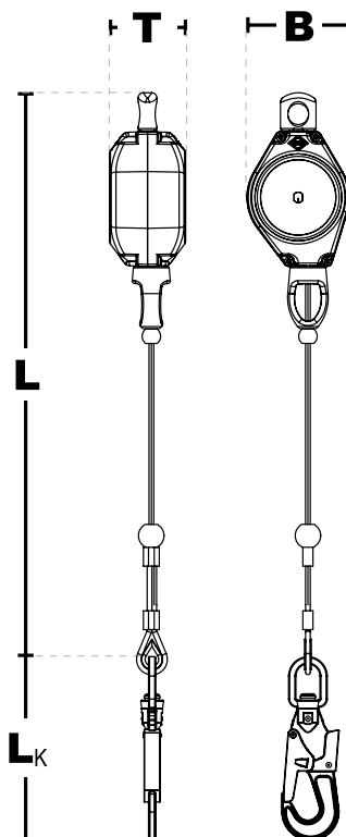
IKV 21 (EN 362:2004-T) with fall indicator
