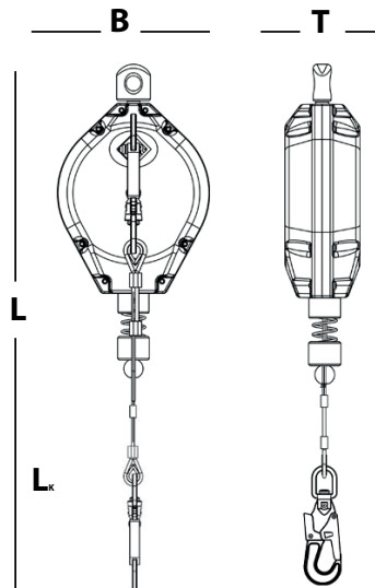
IKV 33 (ANSI Z.359.1-2007; CSA Z259.12-2011) mit Fallanzeiger
